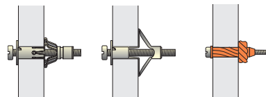
Kotva kovová „Molly“ Dutinová kovová hmoždinka - HM Plastová uzlovací hmoždinka
